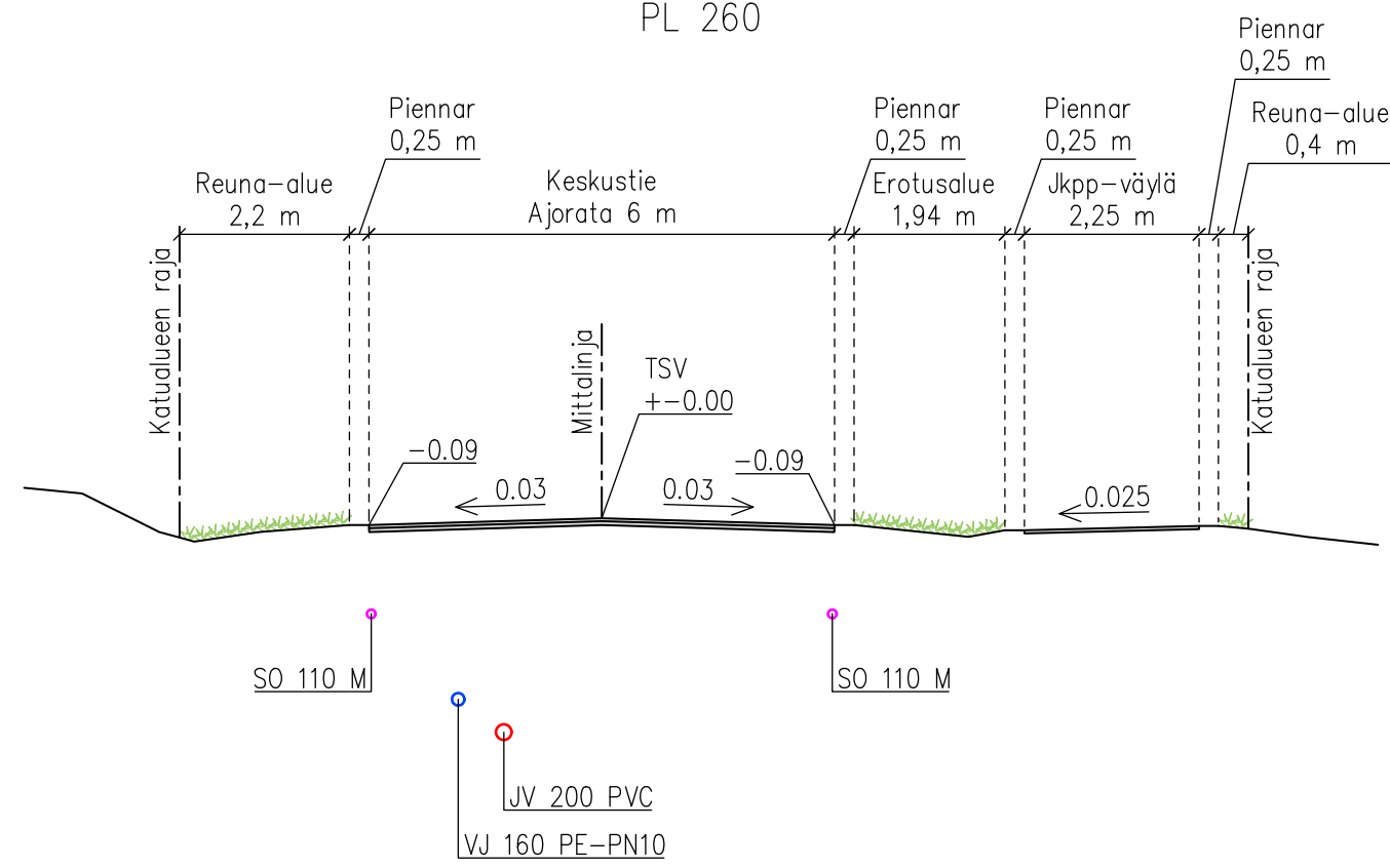
Tyypipoikkileikkaus PL 260
