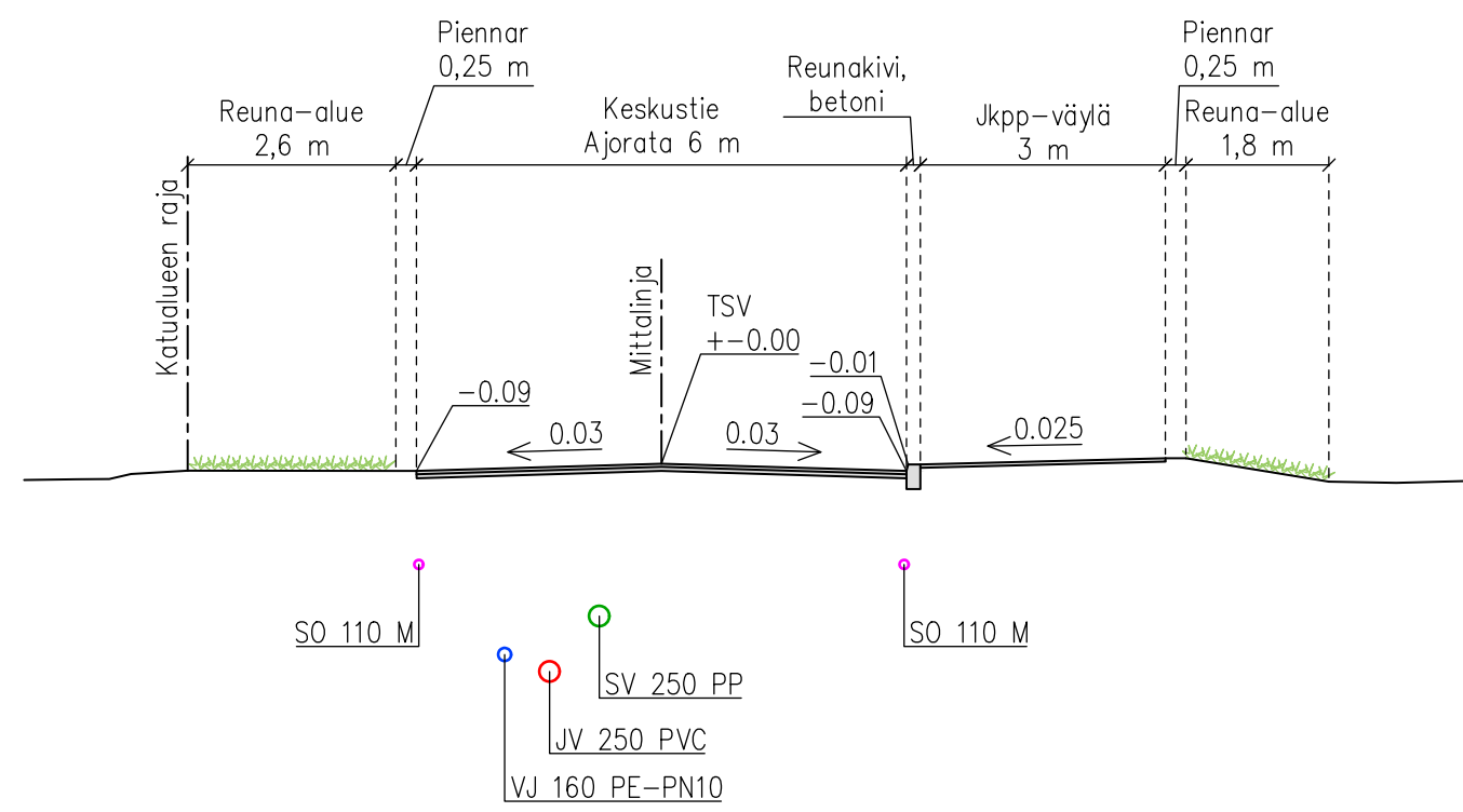
Tyypipoikkileikkaus PL 170
