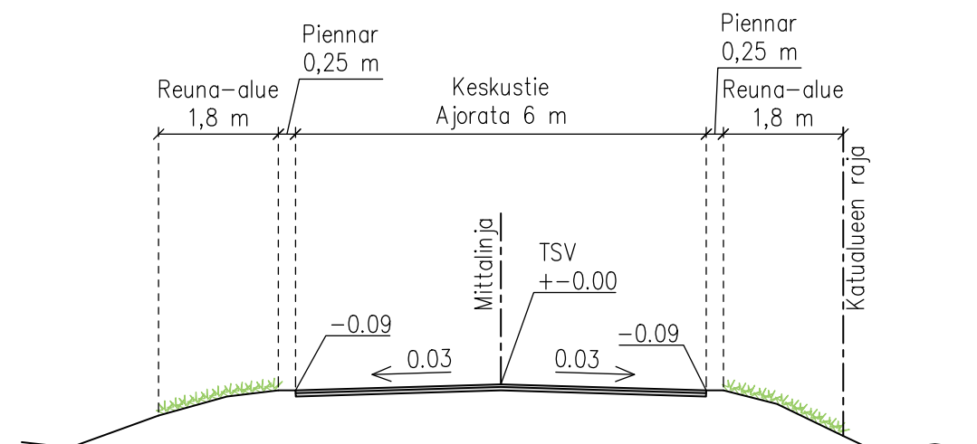
Tyypipoikkileikkaus PL 350
